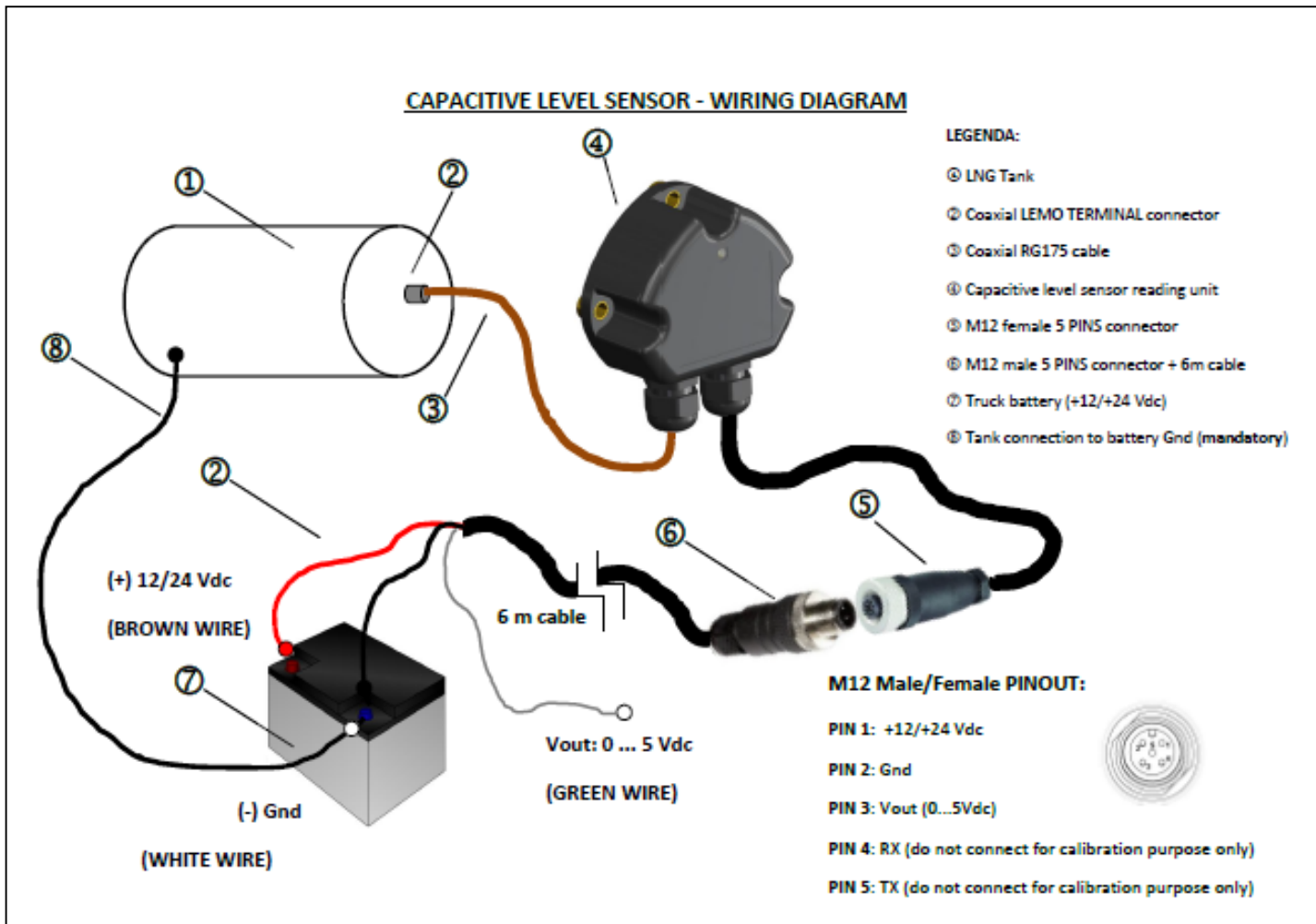
Figura 1 - Diagramma dei collegamenti.
